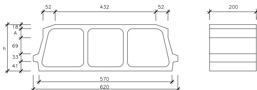
SECCION TRANSVERSAL
